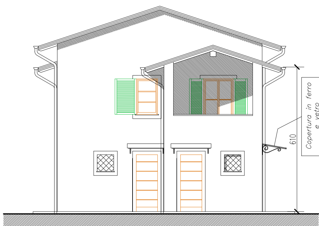
PROSPETTO NORD
