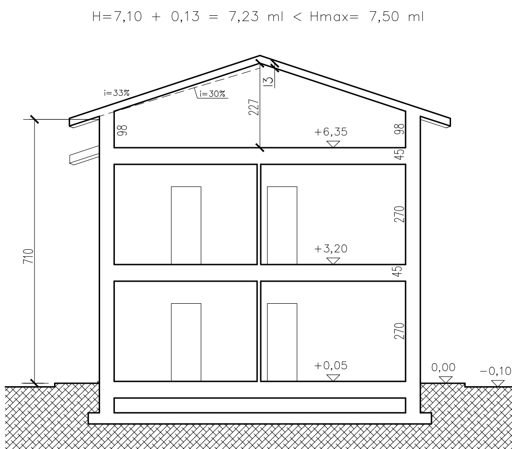
SEZIONE A-A SCALA 1:100
