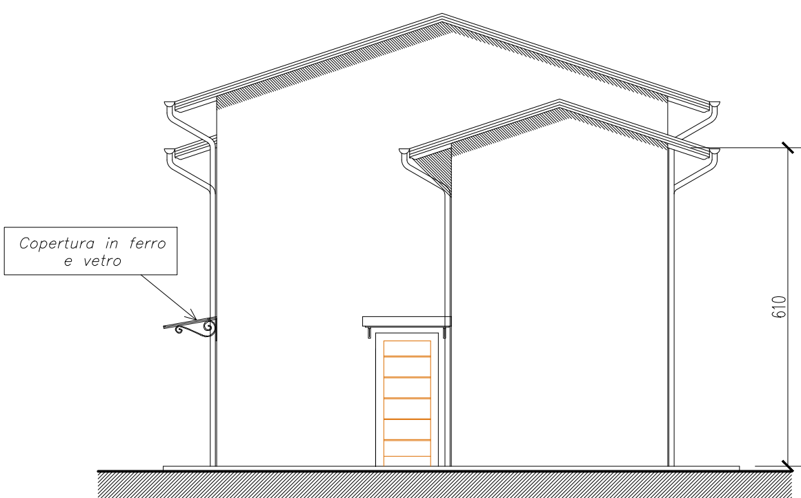
PROSPETTO SUD
