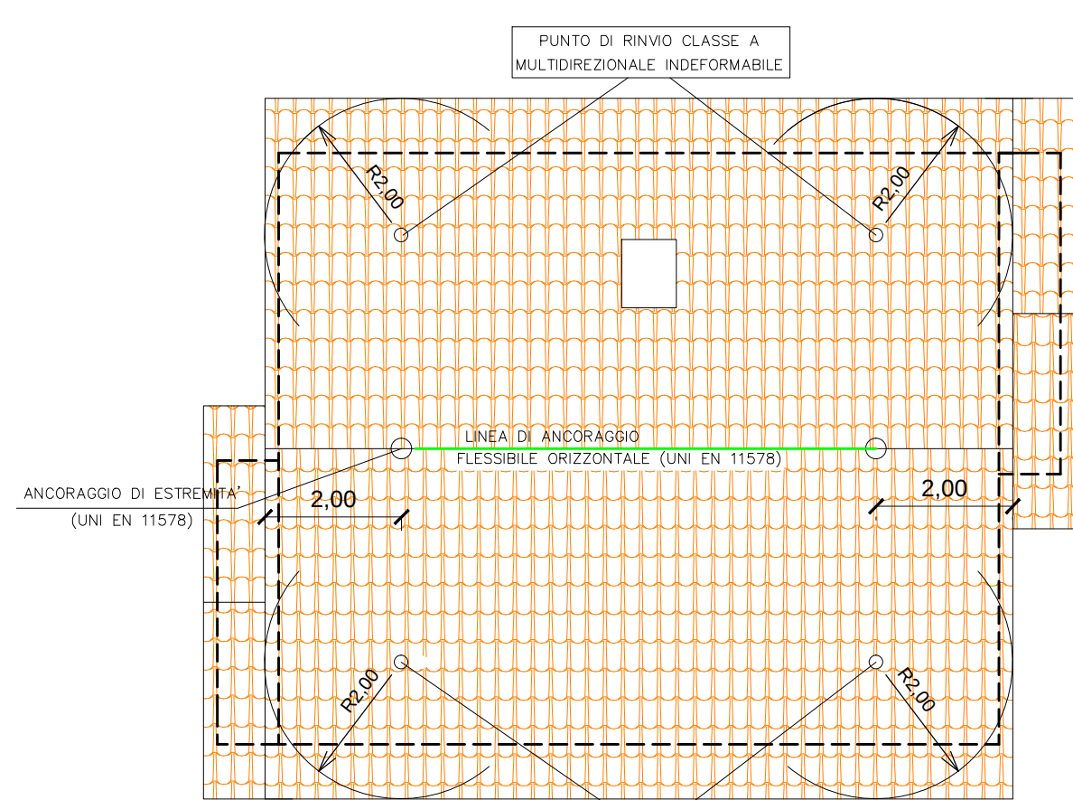
COPERTURA SCALA 1:100
