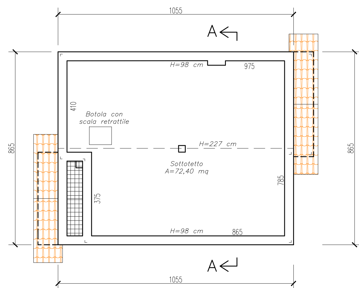
SOTTOTETTO SCALA 1:100
