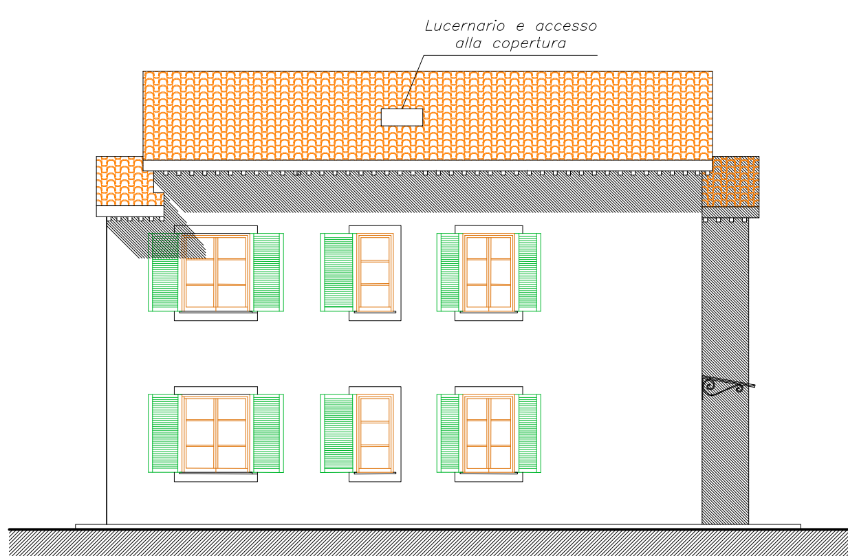
PROSPETTO OVEST
