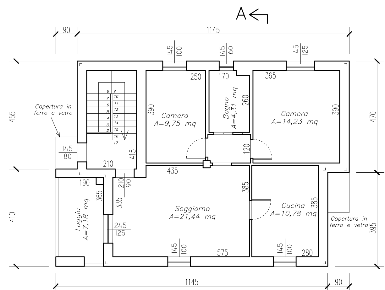
PIANO PRIMO SCALA 1:100
